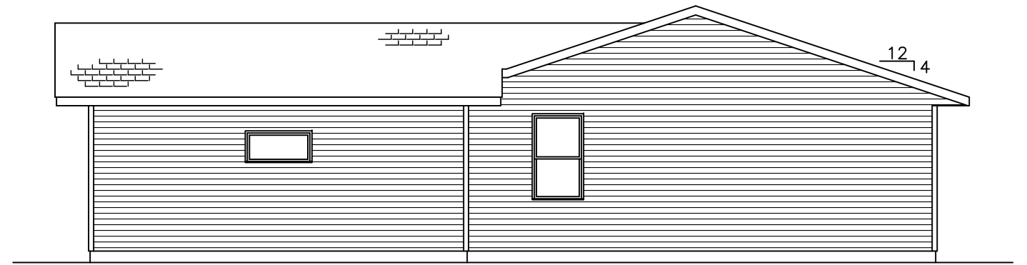
END ELEVATION
