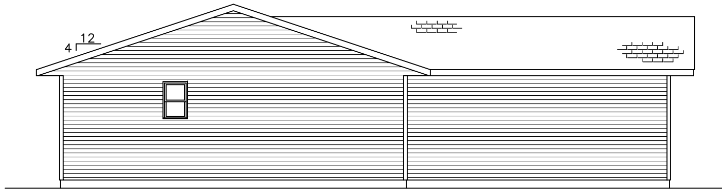
END ELEVATION
