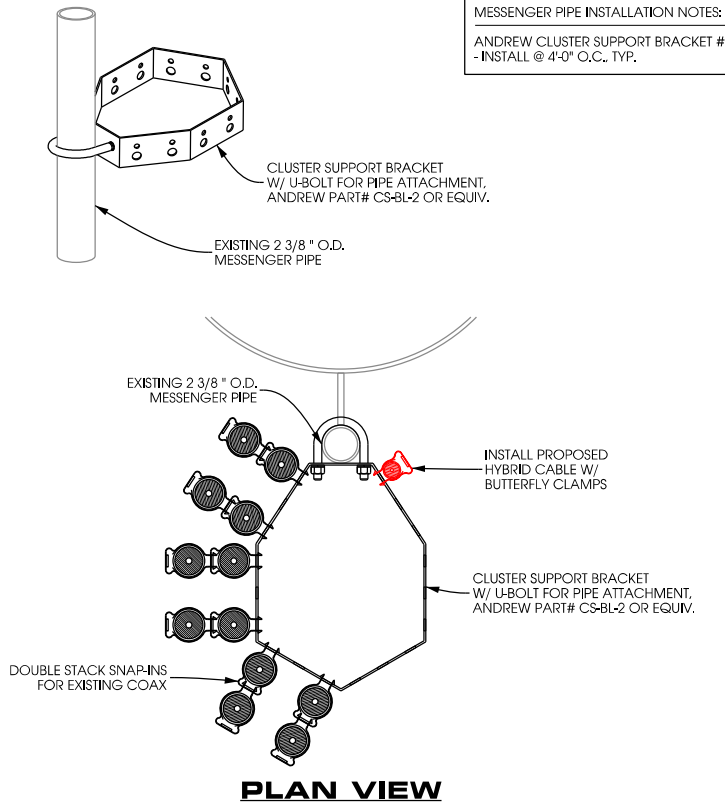
E CLUSTER BRACKET DETAILS A-5 SCALE: 11 x 17 - 1" = 1'-0" 22 x 34 - 1" = 0'-6"
