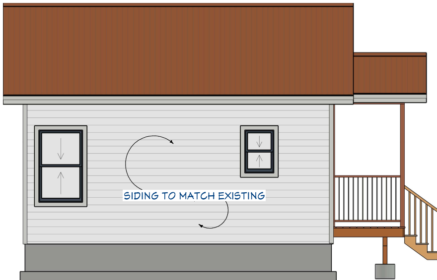
Elevation 3
