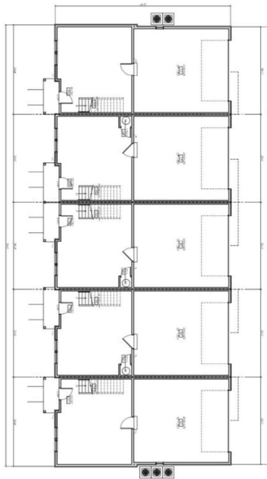
SOLEX - LEVEL 1 - 3 STORY SCALE: 1/8" = 1'-0"
