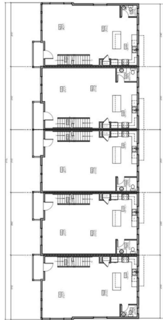
2 SOLEX - LEVEL 2 - 3 STORY SCALE: 1/8" = 1'-0"
