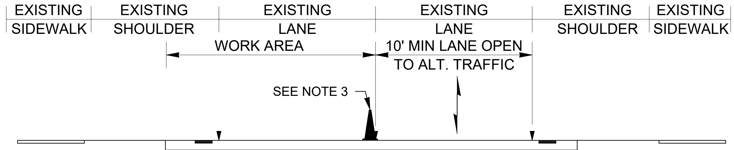
SECTION A-A
