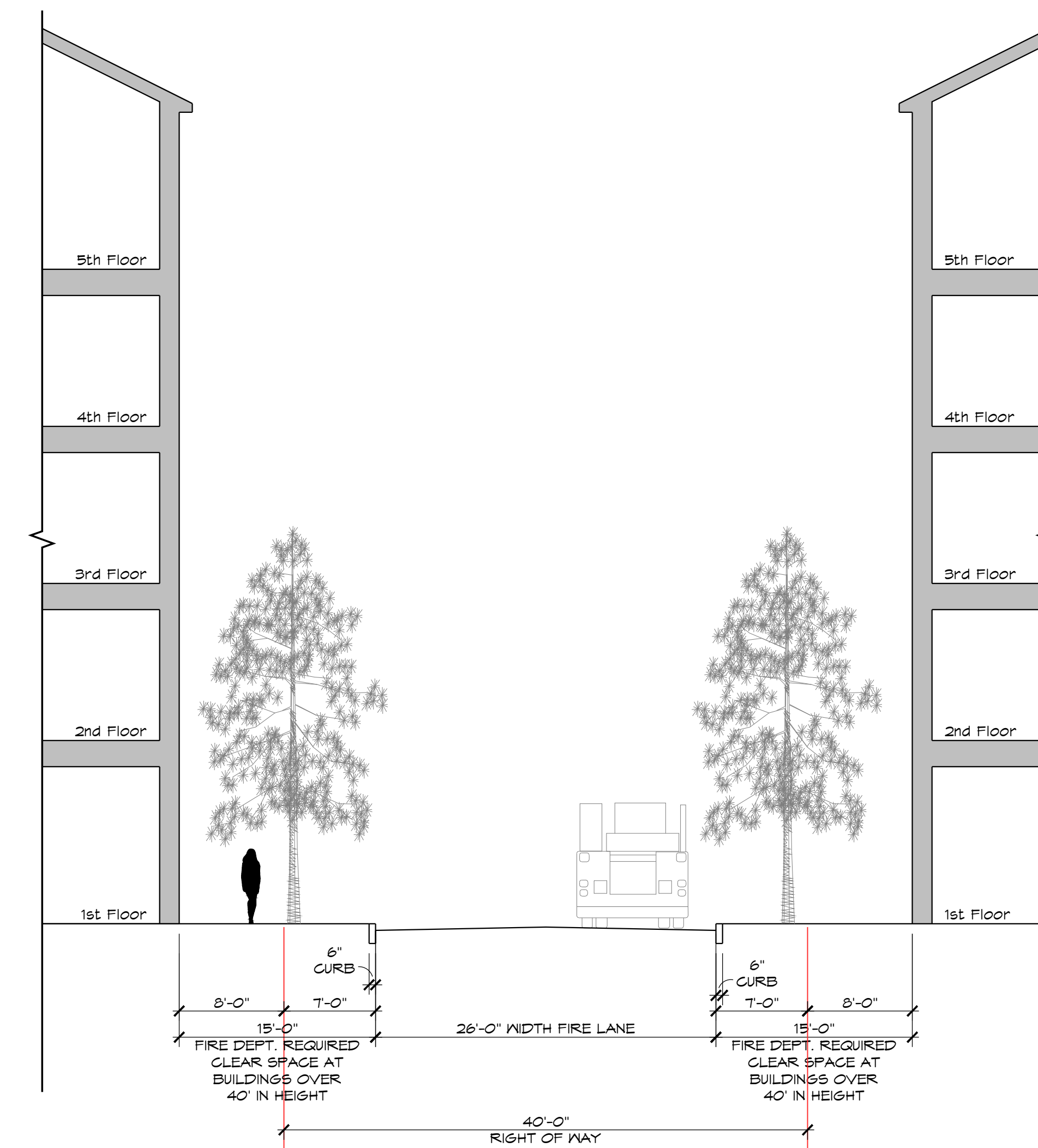
TYP. R.O.W.
