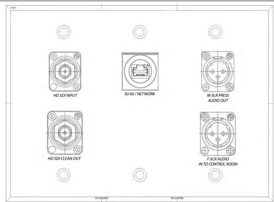
Press Plate
