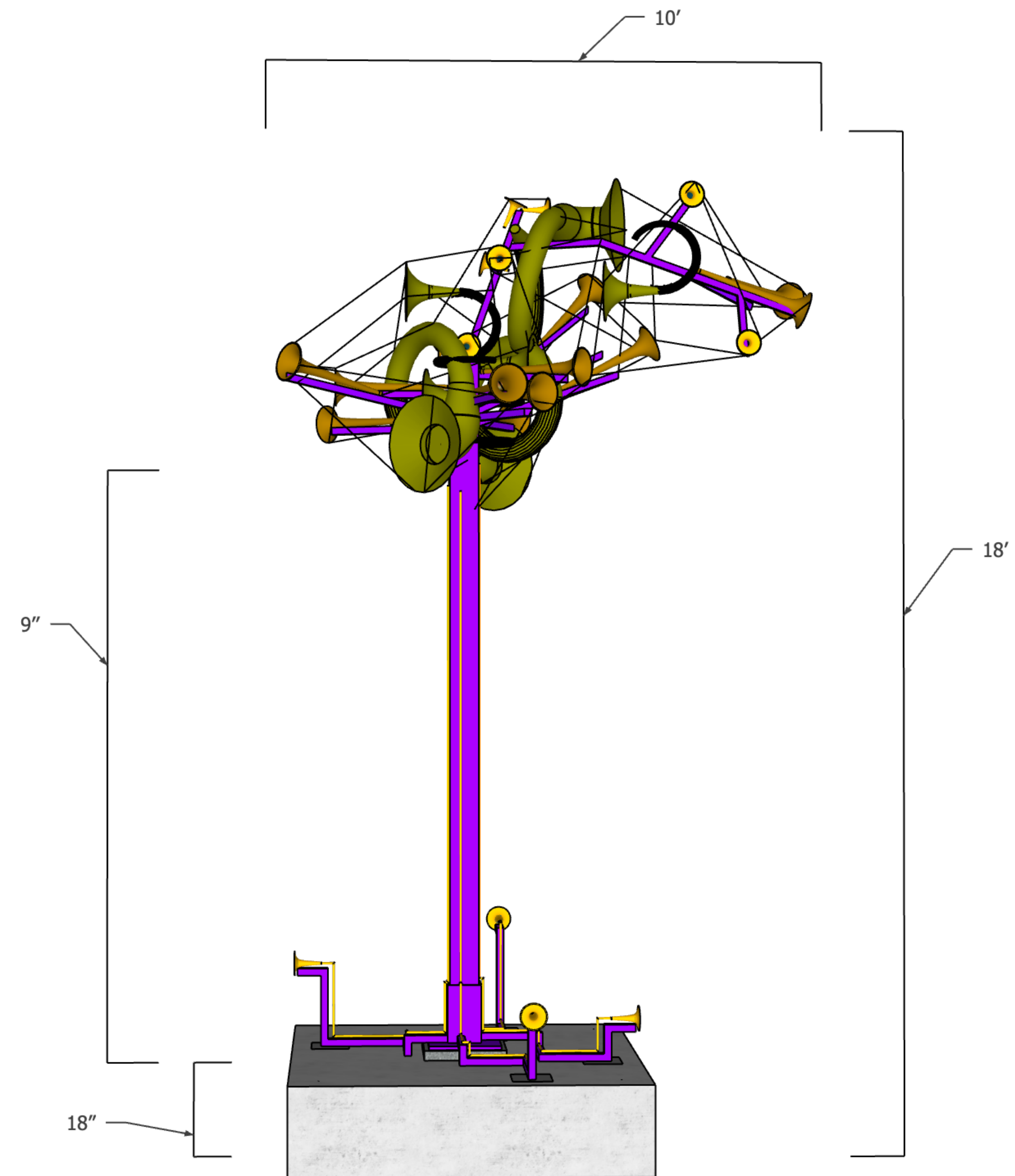
Dimensions
