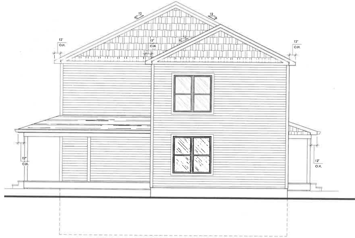
SIDE ELEVATION 2 3 Scale: 1/4" = 1'-0" A3.0
