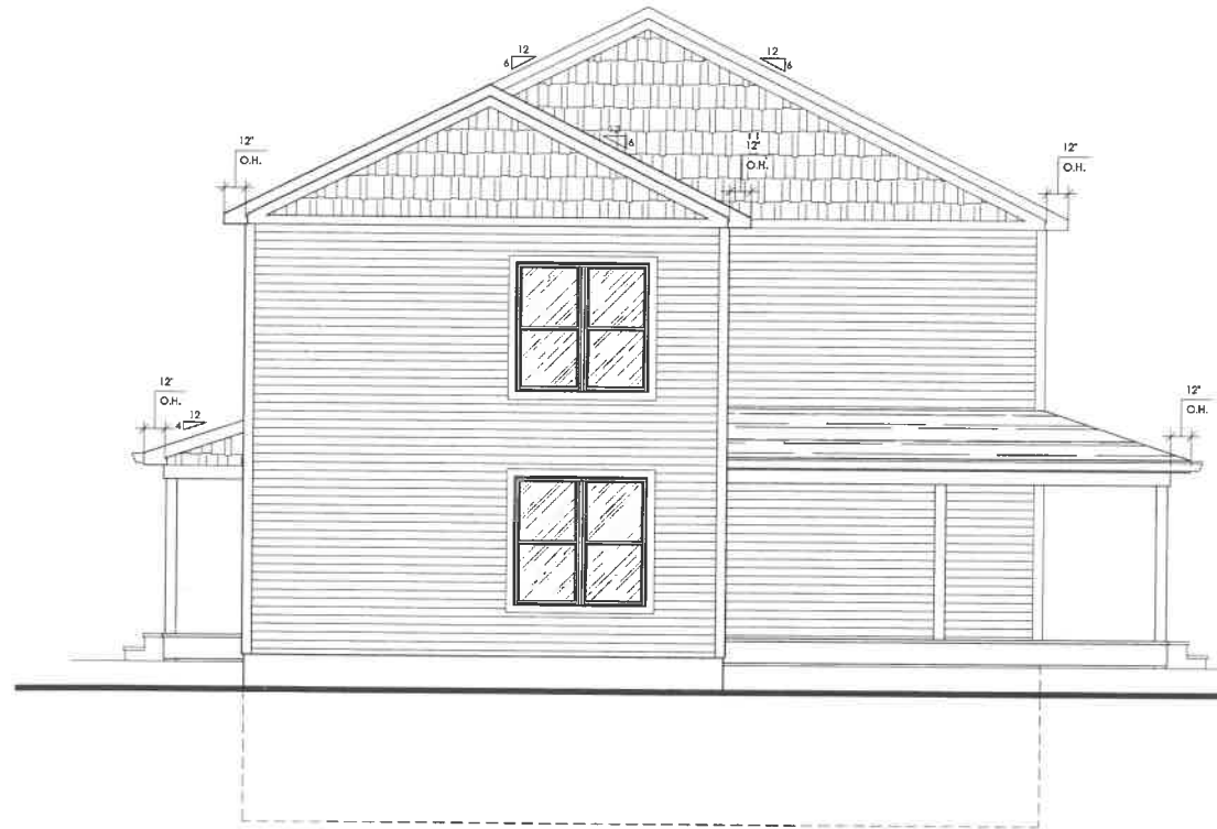
SIDE ELEVATION 1 1 Scale: 1/4" = 1'-0" A3.0
