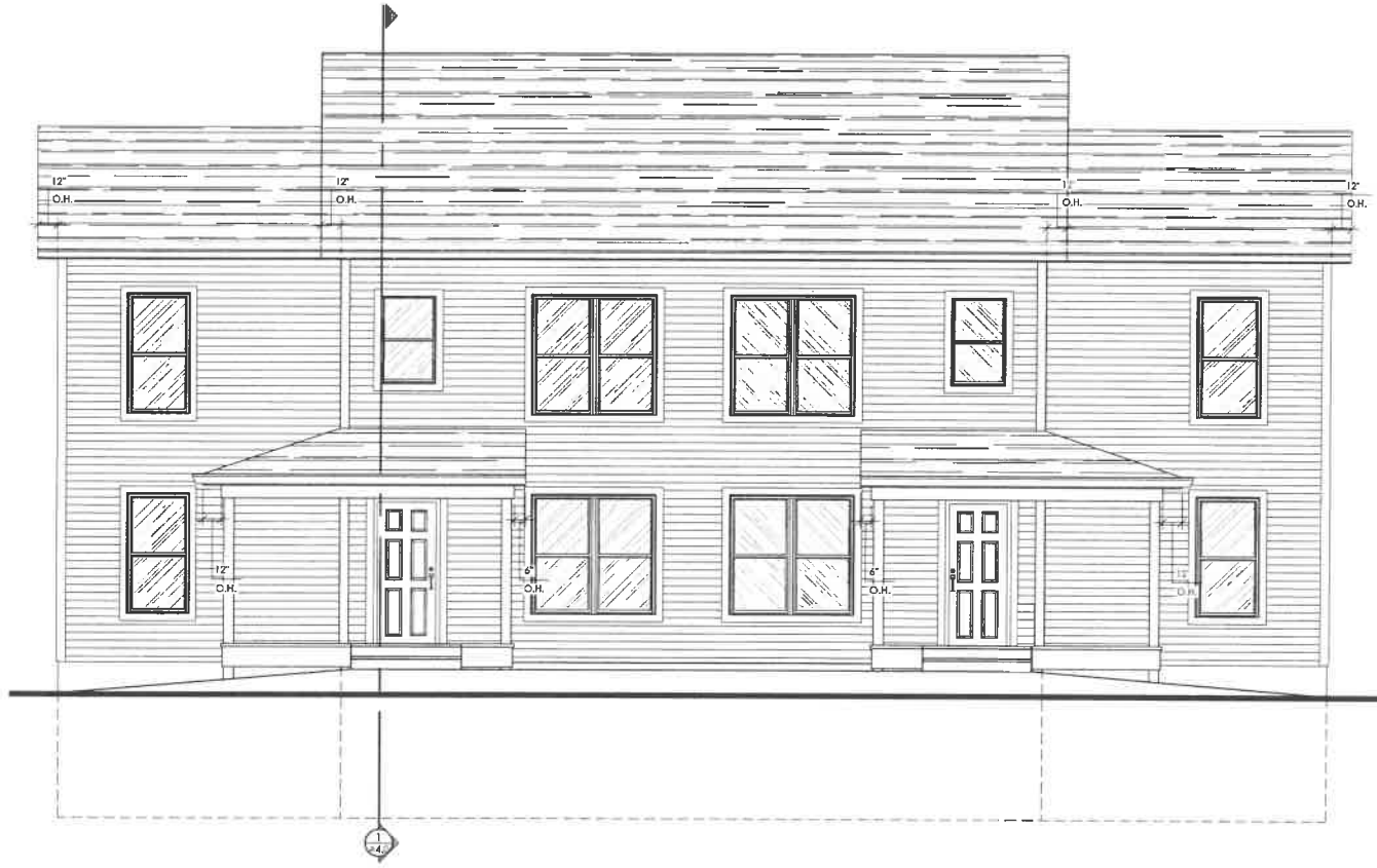
FRONT ELEVATION 4 Scale: 1/4" = 1'-0" A3.0
