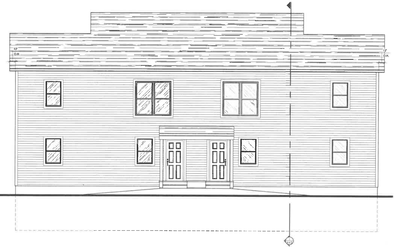
REAR ELEVATION 2 Scale: 1/4" = 1'-0" A3.0
