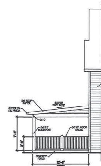
D 1 RIGHT SIDE ELEVATION SCALE: 1/8" = 1'-0"
