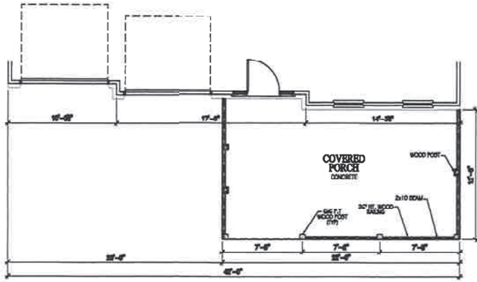
A 1 FLOOR PLAN SCALE: 1/8" = 1'-0"
