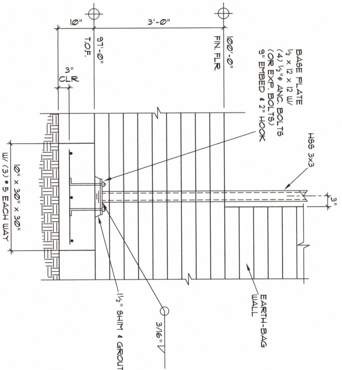
14 SCALE: 3/4"=1'-0"
