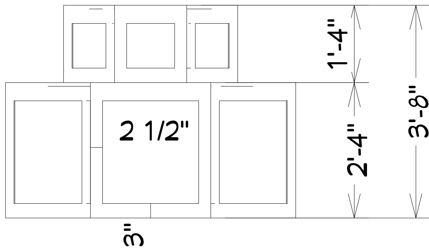
Elevation 1
