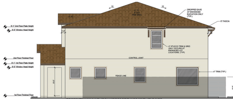
RIGHT ELEVATION - SCL - A SCALE: 1/8\"/>
