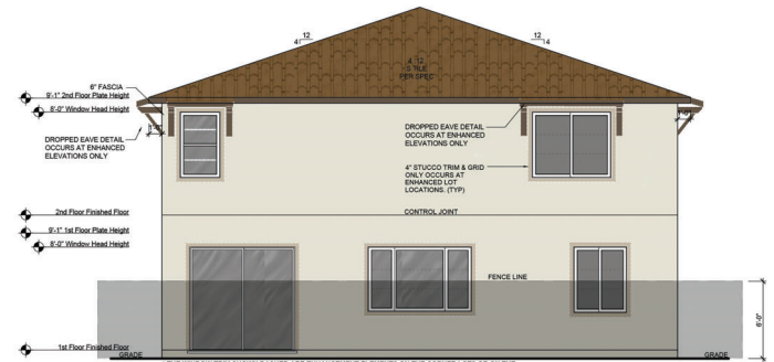
REAR ELEVATION - SCL - A SCALE: 1/8\"/>
