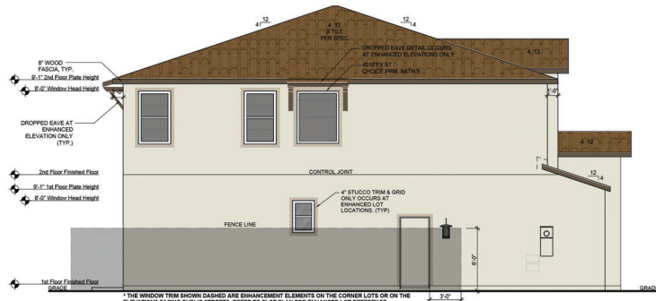
LEFT ELEVATION - SCL - A SCALE: 1/8\"/>
