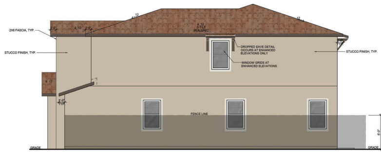
RIGHT ELEVATION - SCL - A SCALE: 1/8\"/>
