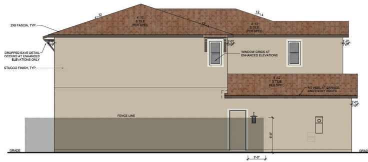
LEFT ELEVATION - SCL - A SCALE: 1/8\"/>
