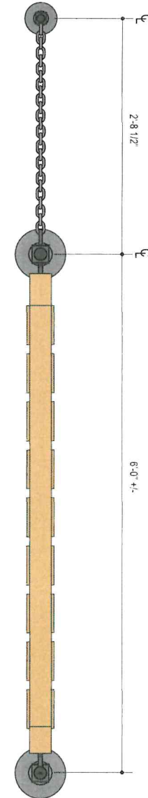
2 SIDE DETAIL SCALE: 1" = 1'
