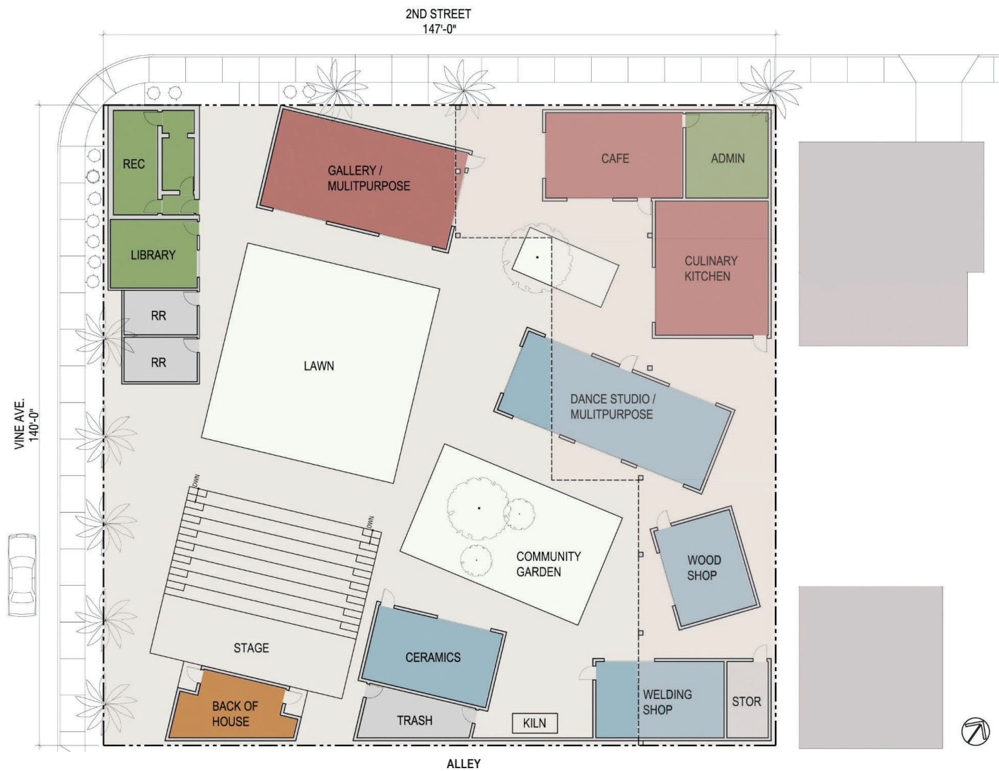
SITE PLAN: Option 1
