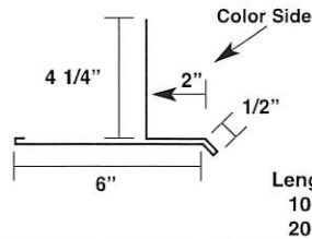
Eave Trim* MDET
