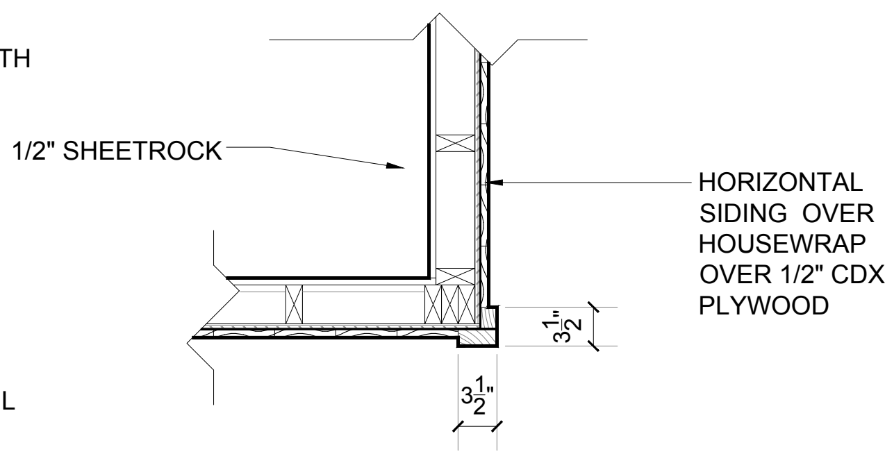
G CORNER DETAIL A2 SCALE: 1"=1'-0"
