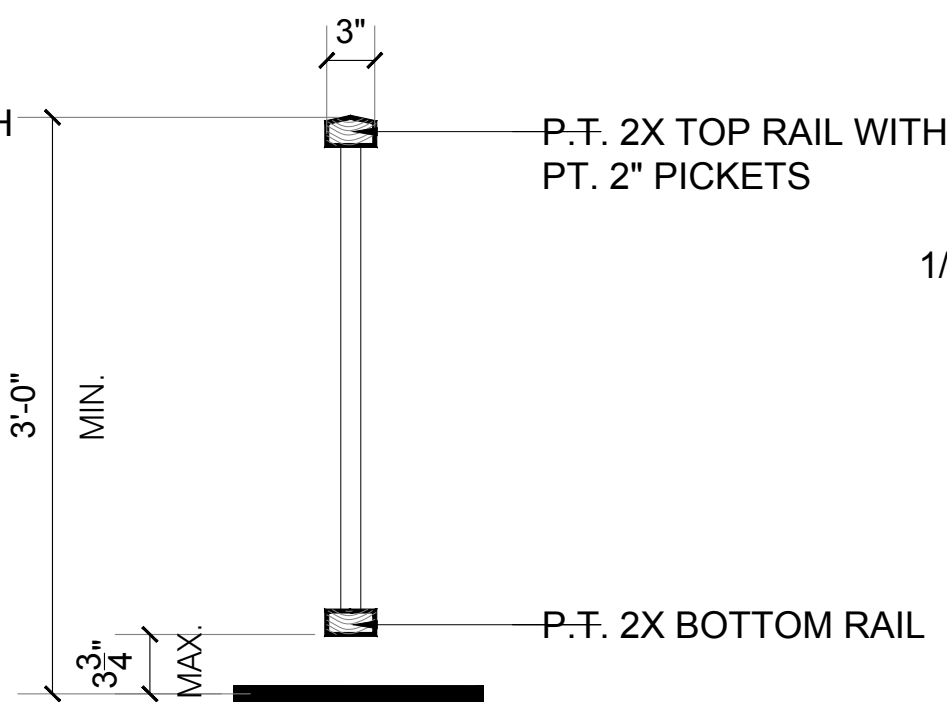
F GUARDRAIL DETAIL A2 SCALE: 1"=1'-0"
