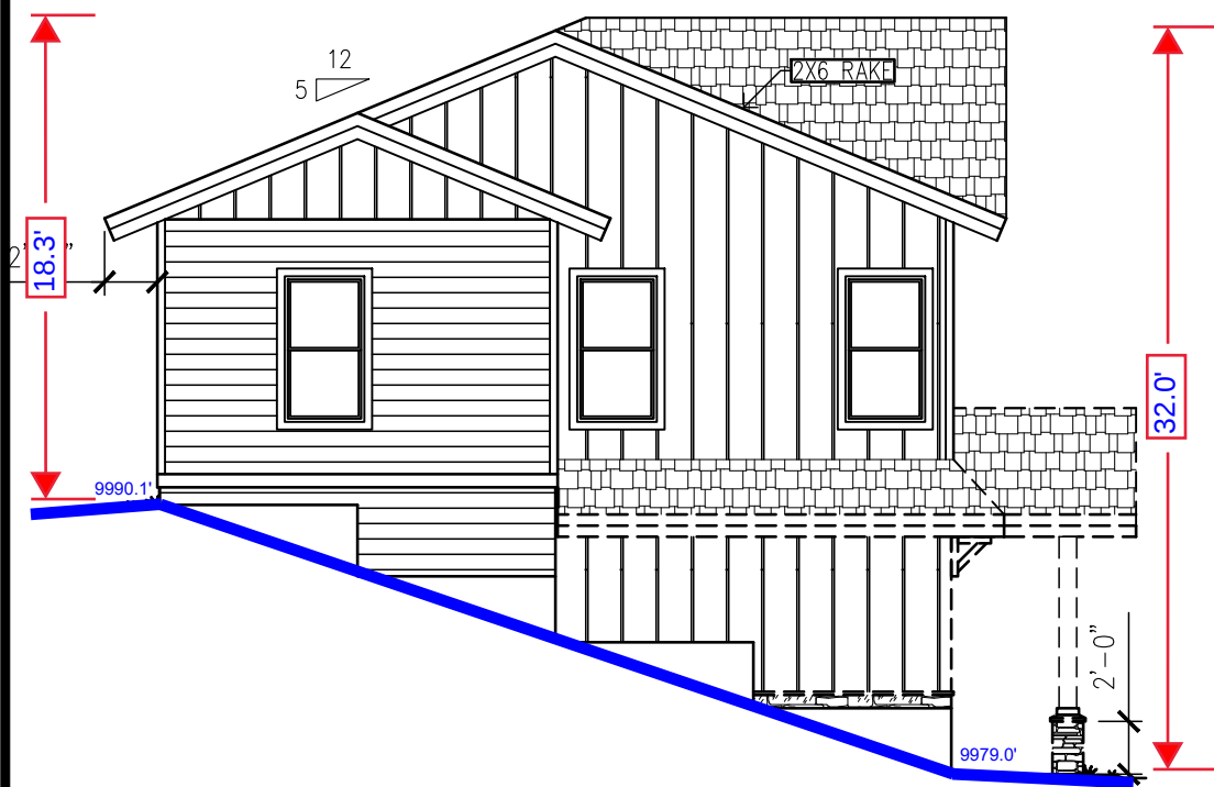
LEFT
